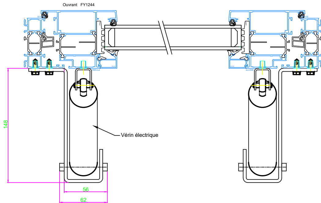
Coupe horizontale BB
